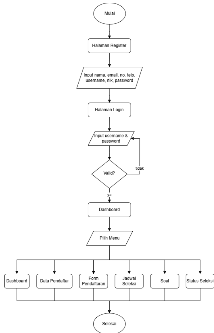
Gambar 3.3 Flowchart Pendaftar
